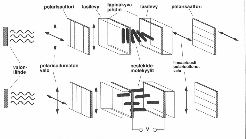
Kuva 2: Kiertonemaattisen nestekidenäytön toimintaperiaate. Ylempänä on nestekidenäytön "kirkas tila", alempana "pimeä tila".
