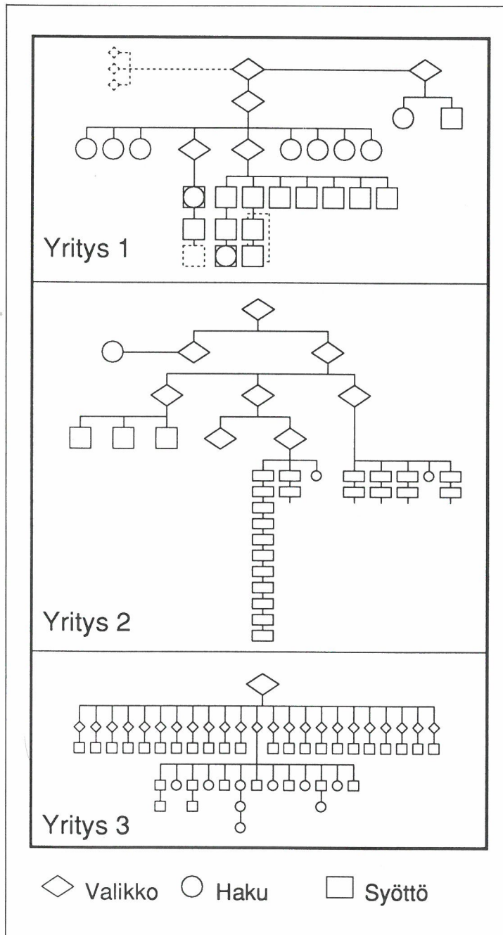
Kuva 4: Yritysten tietojärjestelmien rakenteiden vertailu.
