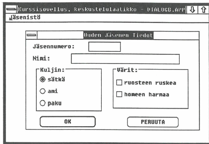
Kuva 5: Rättäriklubisovelluksen keskusteluikkuna.
