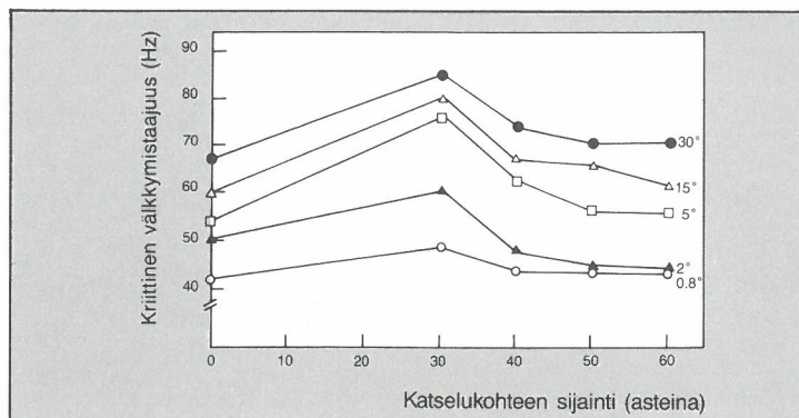
Kuva 1. Keskiarvot (N/6) kriittisestä välkymistaajuudesta. Parametrinä katselukohteen koko ja vaaka-akselina katselukohteen sijainti asteina (Bauer et al 1983. 31–33).
