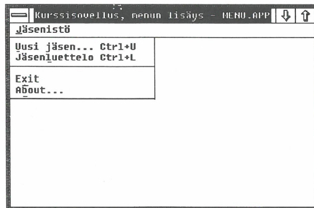
Kuva 3: Esimerkissovelluksen valikkorakenne.
