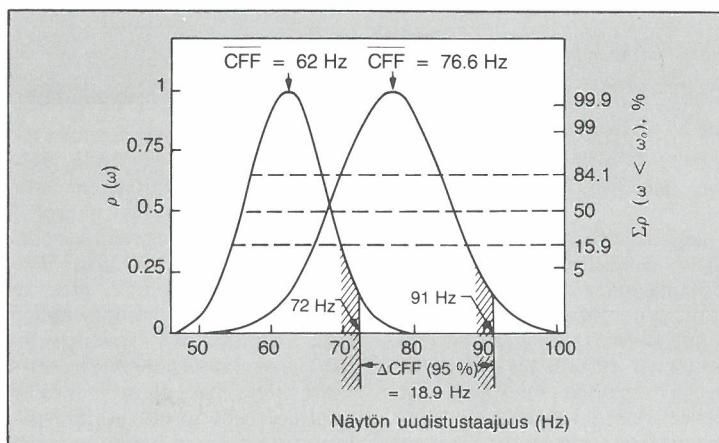
Kuva 2. Kriittisen välkymistaajuuden jakaumat hitaalle (vasemmanpuoleinen jakauma) ja nopealle (oikeanpuoleinen jakauma) fosforille 80 cd/mFD luminanssille (Bauer 1987, 29–32).
