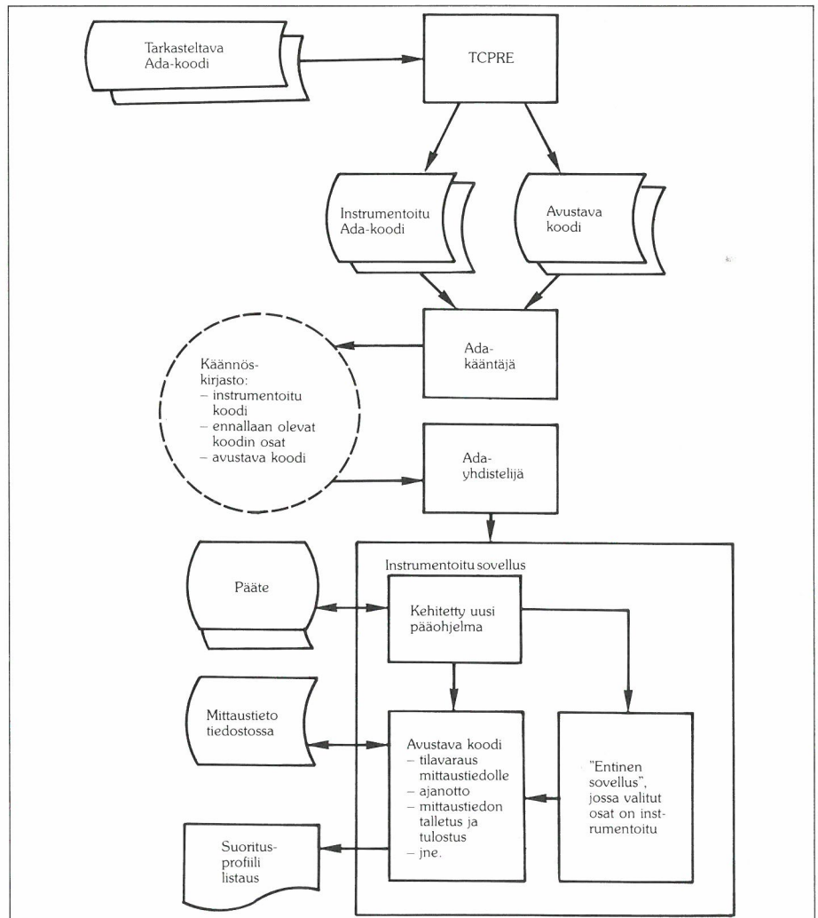
Kuva 2: TCMON-järjestelmän rakenne
