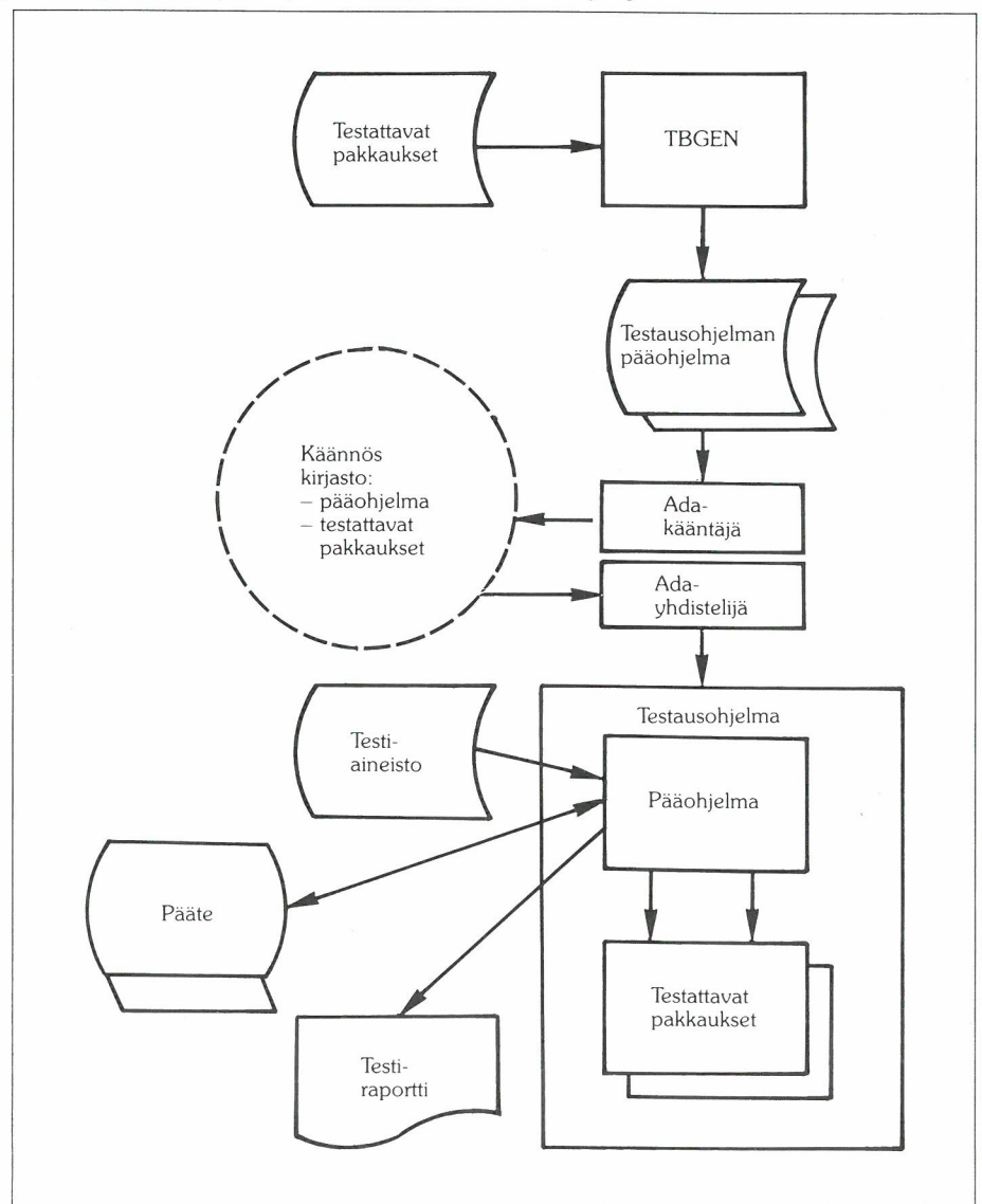
Kuva 1: TBGEN-järjestelmän rakenne
