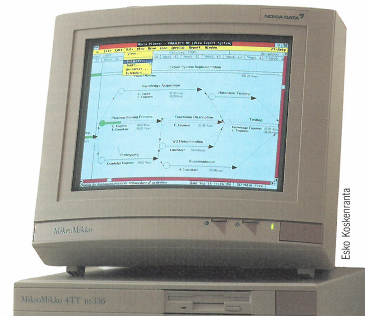
Kuva 2. Tyypillinen Planner-näkymä.
