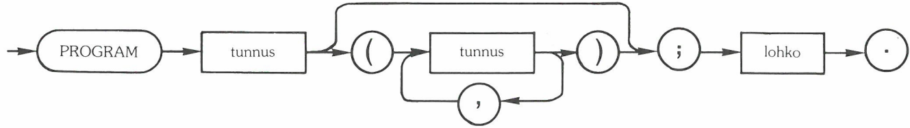
Pascal-ohjelman rakenne
