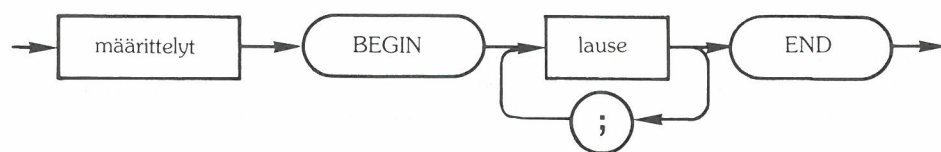
Ohjelmalohkon rakenne
